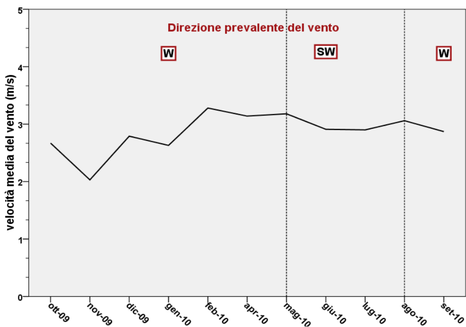
Figura 4.2.1. Andamento di temperatura, precipitazioni (a) e ventosità (b) relativi alla stazione meteorologica dell'ARPA di Settefonti nel periodo ottobre 2009-settembre 2010 (W= ovest; SW= sud-ovest)
