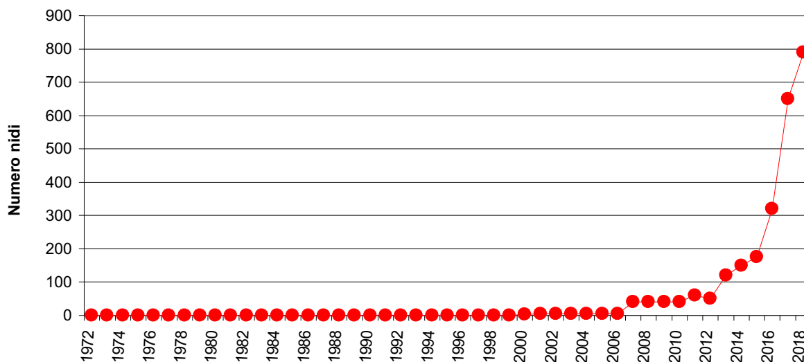
Figura 1.12 - Indice della popolazione di ibis sacro nidificante nelle garzaie della Pianura Padana nord-occidentale censite nell'ambito del programma Garzaie Italia. Ridisegnato da Fasola 2019.
