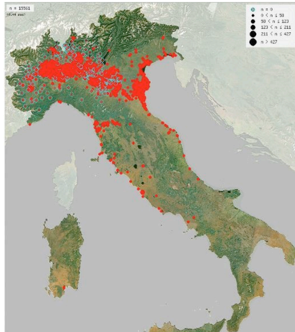
Figura 1.10 - Osservazioni di ibis sacro dal 1990 al gennaio 2018 (N = 15561). (Fonte: Ornitho.it).
