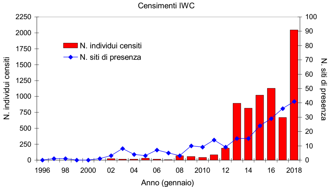
Figura 1.2 - Numero di ibis sacri e numero di siti occupati rilevati durante i censimenti degli uccelli acquatici svernanti nel periodo 1991-2017. I dati di presenza degli ultimi anni di rilevamento sono in corso di verifica, pertanto i totali qui riportati potranno essere oggetto di modifica. Fonte: banca dati ISPRA.
