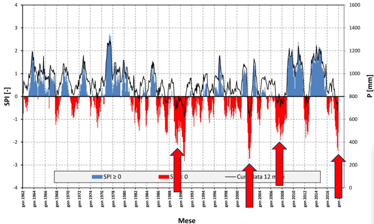
Valori mensili dell'SPI nel 2017 calcolati per l'Italia alle aggregazioni temporali di 1, 2, 3, 6, 9, 12, 24 e 48 mesi, rispetto al periodo 1961 – 2017.
