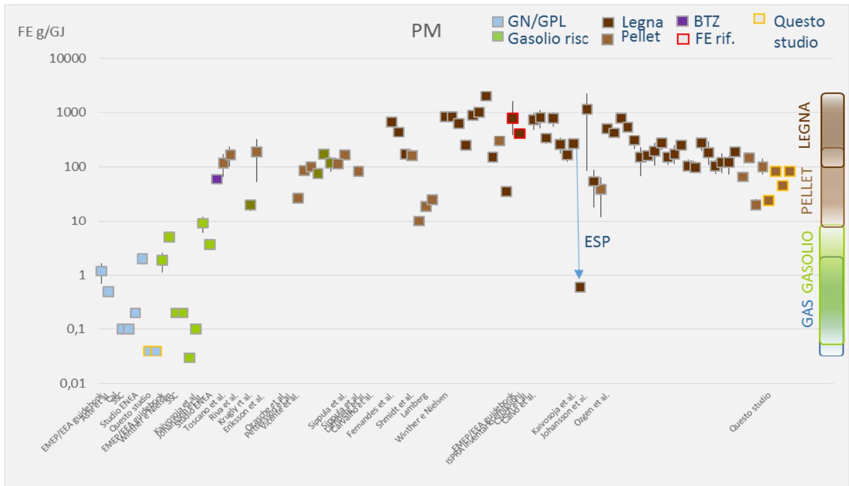
Figura 15 Fattori di emissione per il PM reperiti in letteratura o direttamente ricavati nella sperimentazione di questo studio (ESP: riduzione ottenuta su impianto di grande taglia dotato di filtro elettrostatico)
