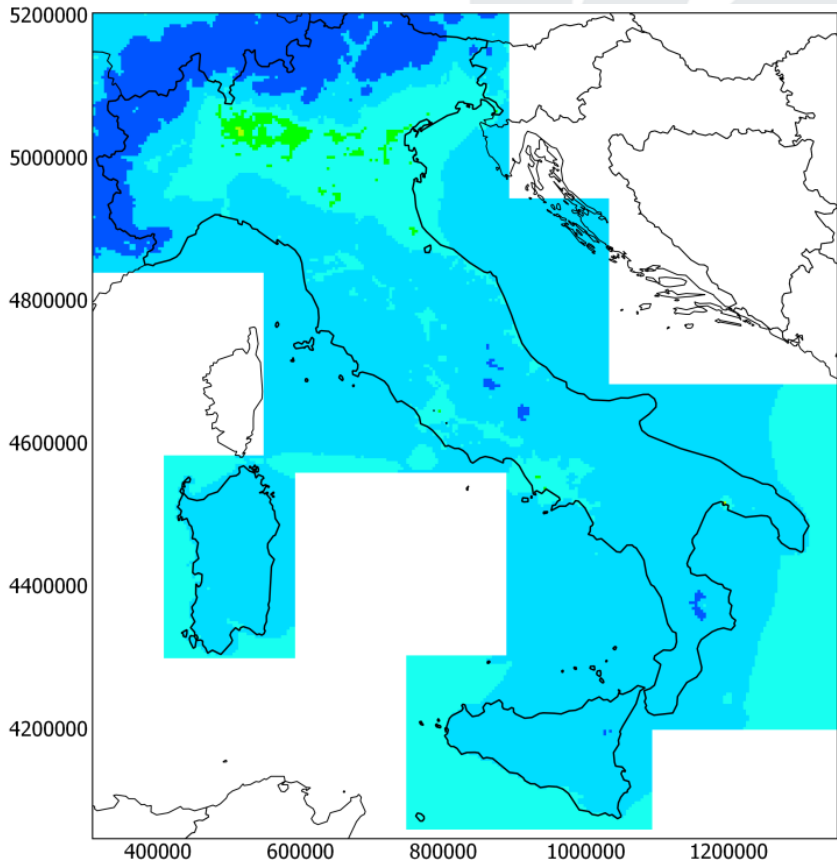
2030 Scenario NEC misure aggiuntive (2018)
